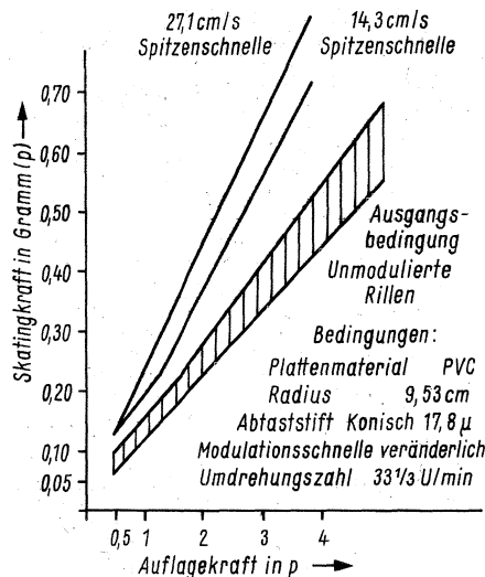
Bild 6. Typische Auswirkung der Skatingkraft in Abhängigkeit von der Auflagekraft (modulierte Rillen, konischer Abtaststift)
