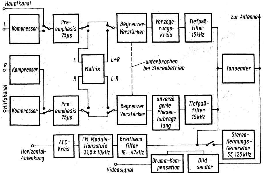
Bild 8. Aufbau eines Zweikanal/Stereo-Senders nach dem FM-FM-Verfahren
