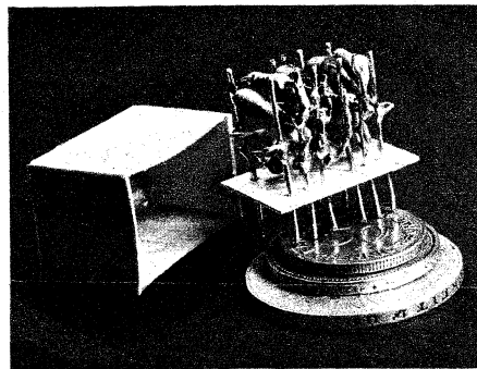
Bild 4. Noch nicht vergossener Modul mit abgenommener Schutzhaube (Aufnahme: Leutmayer)
