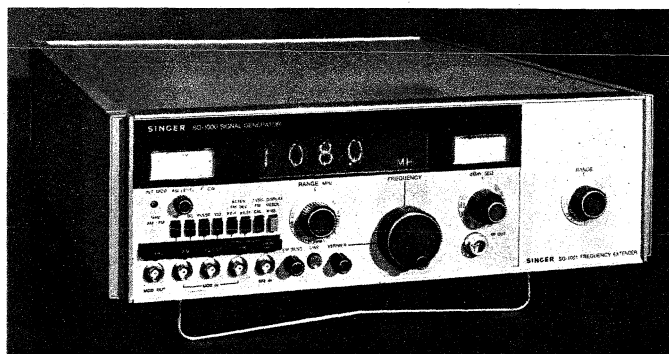
Die digitale Frequenzanzeige gehört u. a. zu den Besonderheiten des Meßsenders SG 1201 von Singer Instrumentation
