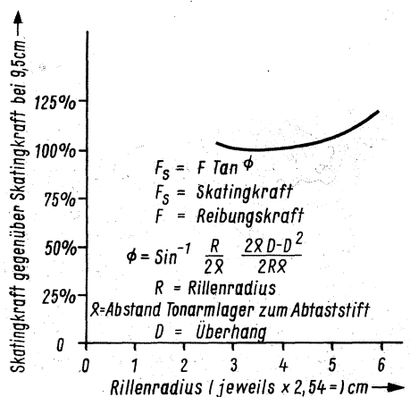
Bild 8. Skatingkraft in Abhängigkeit vom Rillenradius
