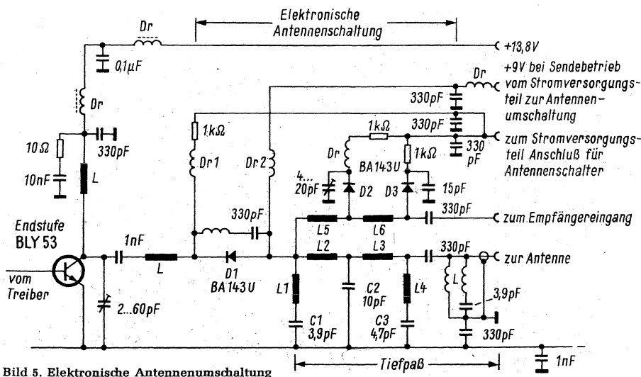
Bild 5. Elektronische Antennenumschaltung
