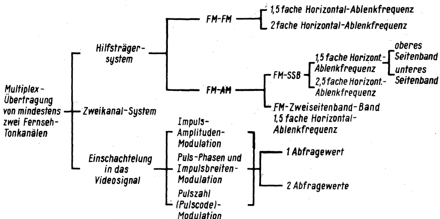
Bild 1. Klassifizierung der zweikanaligen Multiplex-Tonverfahren
